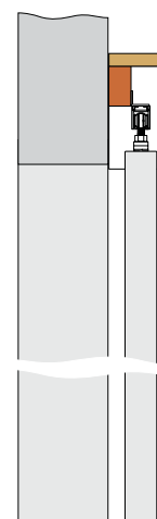
Nástěnný posuvný systém bez obložkové zárubně.
